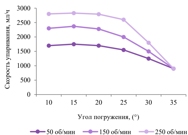
Рисунок 3. Влияния угла погружения на скорость упаривания
