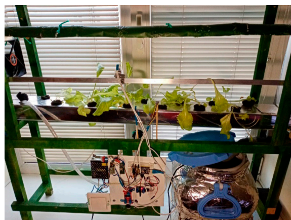
Рисунок 6. Собранный установка гидропоники
