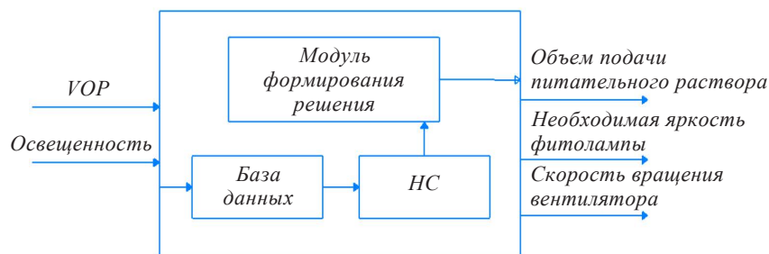
Рисунок 7. Структура регулятора нейронной сети
