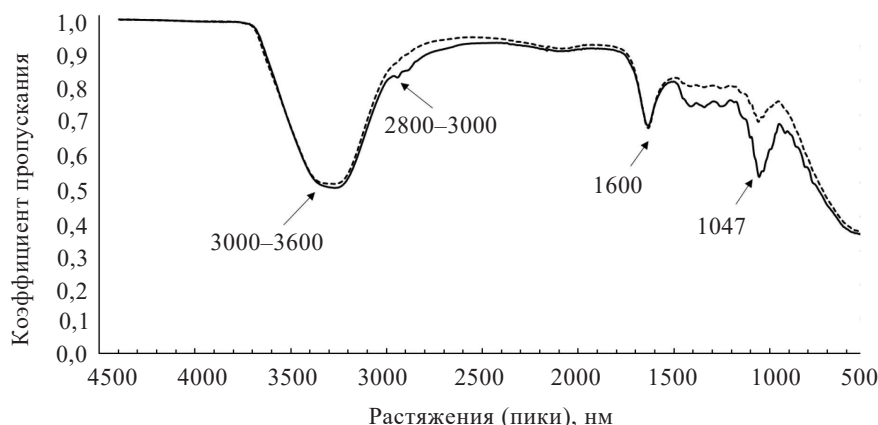
Рисунок 7. FT-IR спектры контрольного образца (пунктирная линия) и предварительно обработанных + высушенных в ИК-сушилке яблочных чипсов толщиной 5 мм (черная линия)
