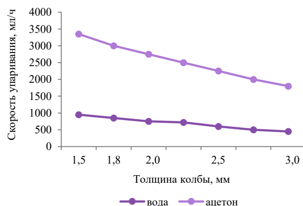
Рисунок 1. Влияние толщины колбы на эффективность упаривания
