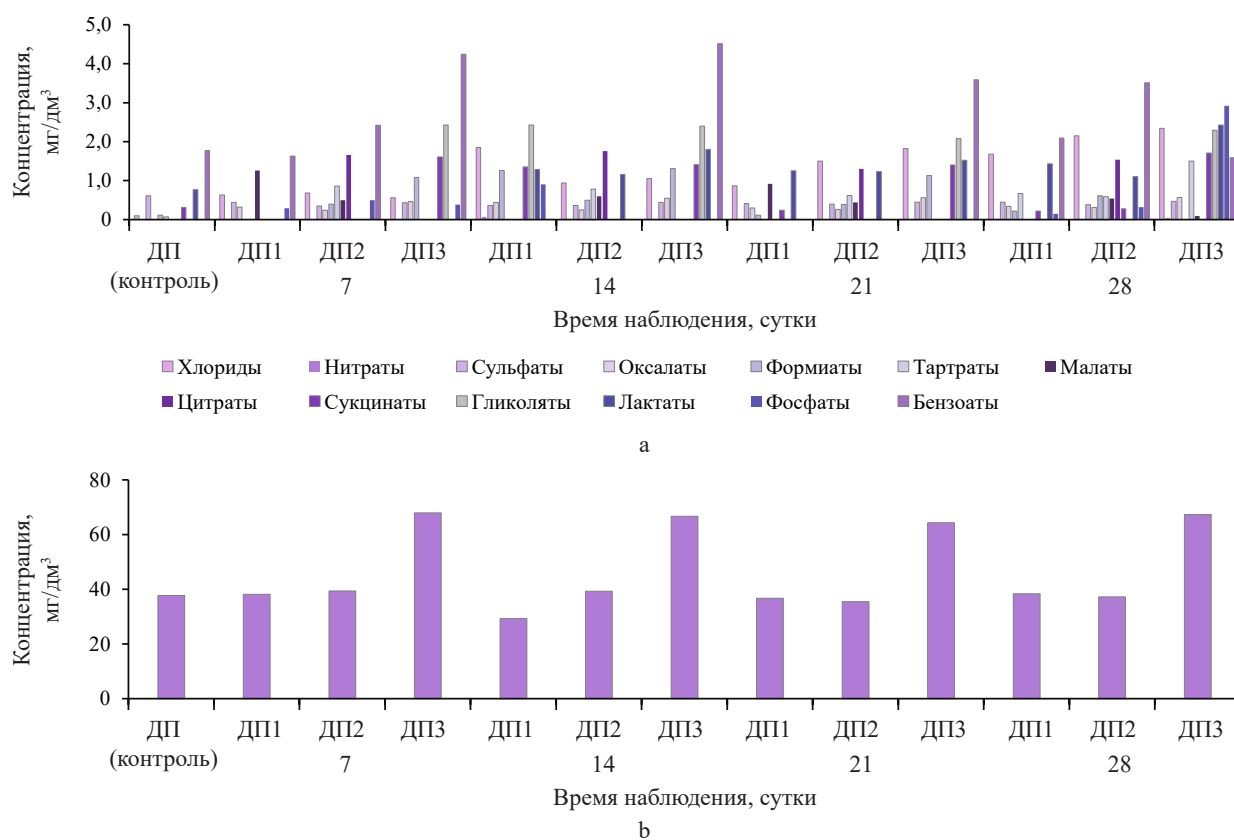
Рисунок 4. Анионный состав модельных образцов зерновых дистиллятов: а – хлориды, нитраты, сульфаты, оксалаты, формиаты, тартраты, малаты, цитраты, сукцинаты, гликоляты, лактаты, фосфаты, бензоаты; б – ацетаты
