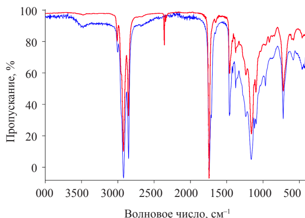
Рисунок 5. ИК-спектр масла без обработки (синяя линия) и после обработки (красная линия)
