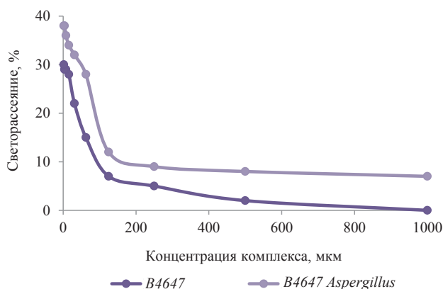
Рисунок 5. Зависимости интенсивности светорассеяния растворов от концентрации комплекса [(\text{NO}_2)_2\text{Pt}^{\text{II}}(\mu\text{-NO}_2)_2\text{Pt}^{\text{II}}(\text{NH}_3)_2]
